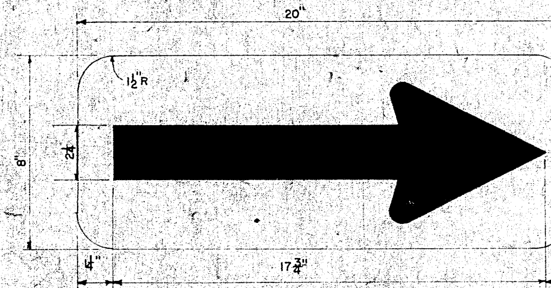
M-9A 20"x8"
