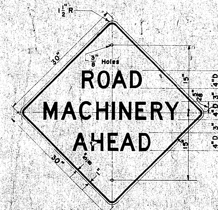
W-147 30"x30"
