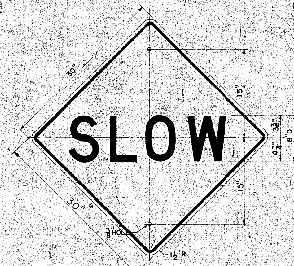
W-155 30"x30"
