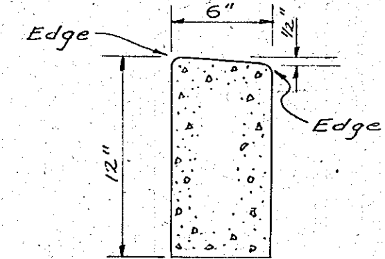
HEADER CURB SCALE: 1/2" = 1'-0"
