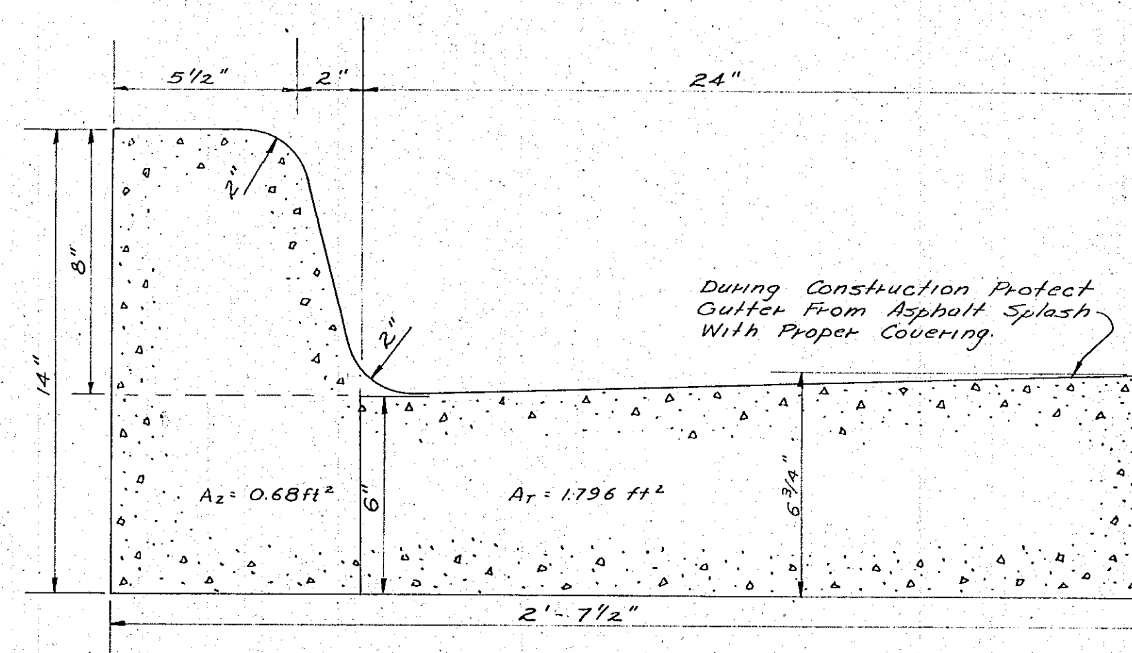
STANDARD CURB SCALE: 3/4" = 1'-0"
