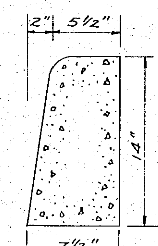
STRAIGHT CURB SCALE: 1/2" = 1'-0"
