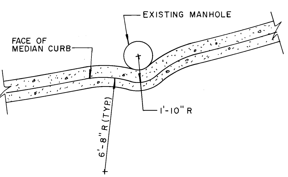
DETAIL A SCALE: \frac{1}{4}" = 1'-0"
