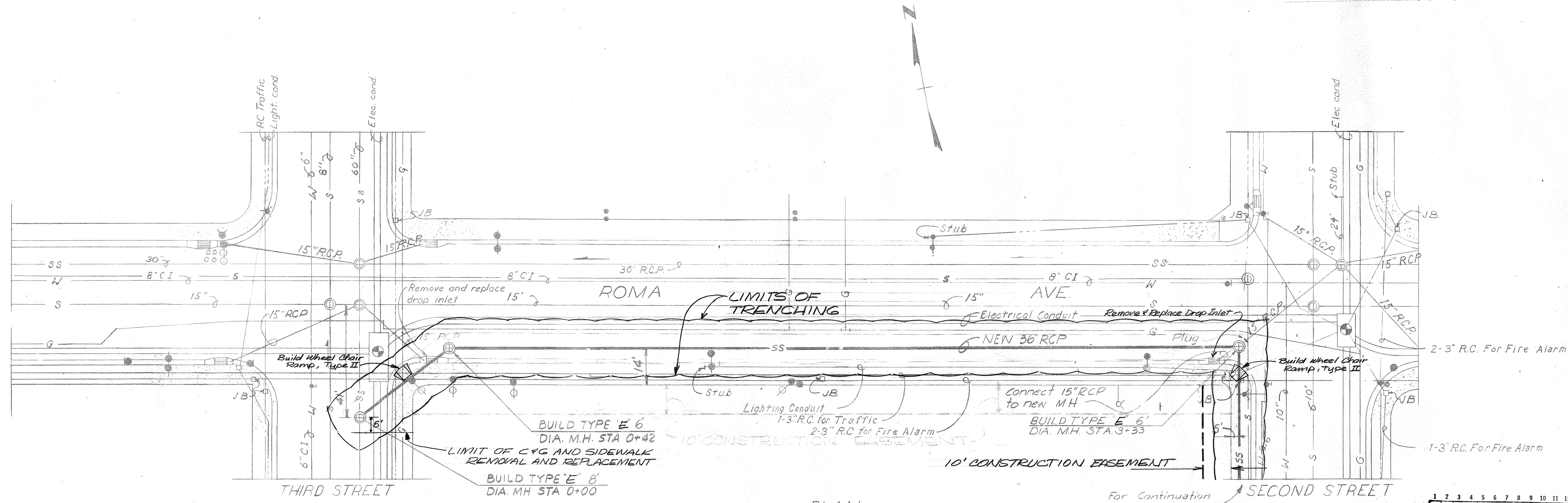
PLAN Scale: 1"=20'
