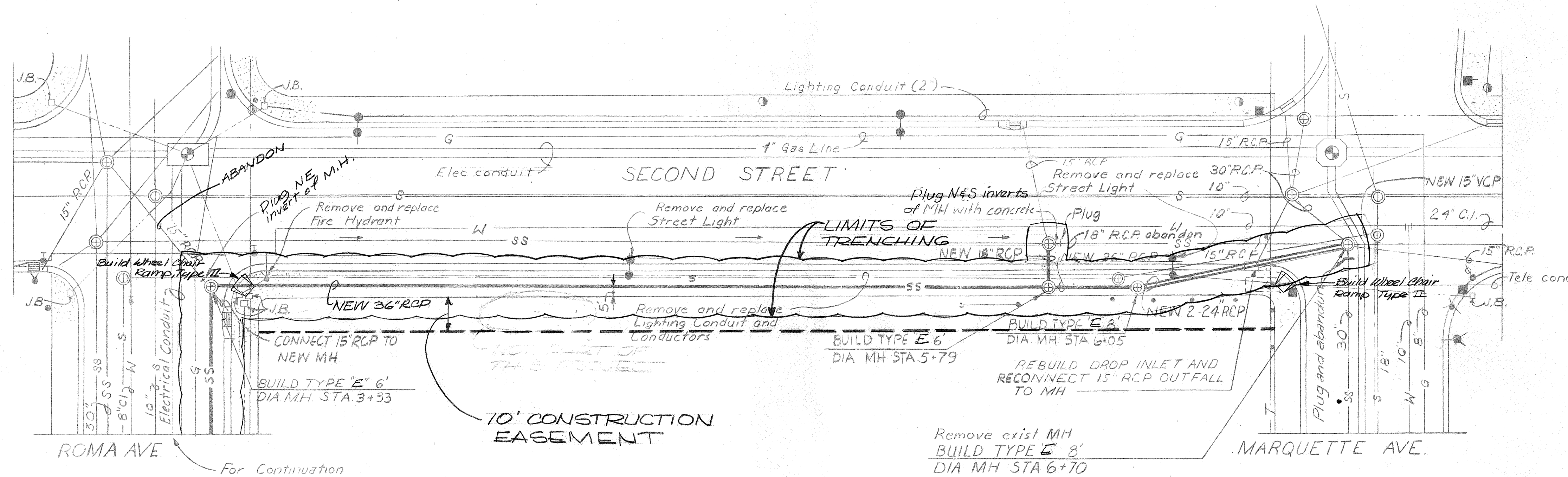
PLAN Scale: 1" = 20'
