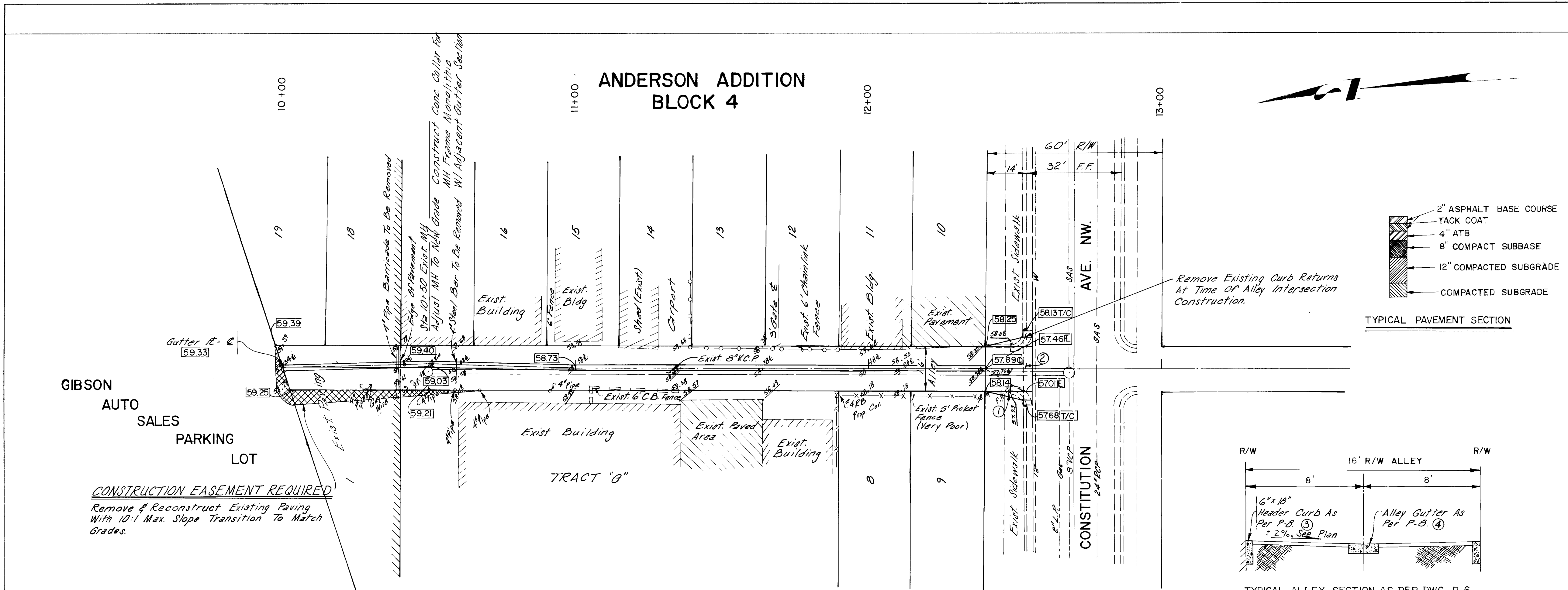
PLAN SCALE: 1" = 20'
