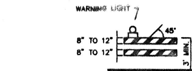
TYPE I BARRICADE
