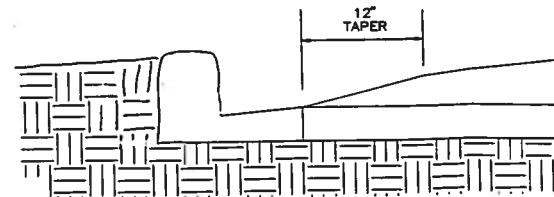
N.T.S. CURB TREATMENT
