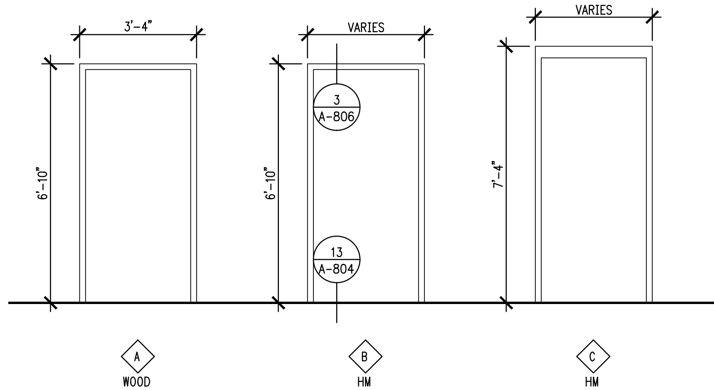
DOOR FRAME TYPES
