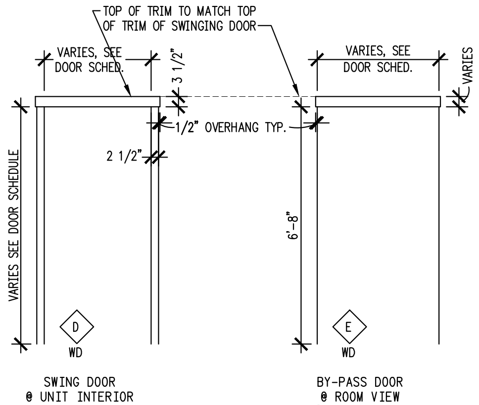
DOOR FRAME TYPES
