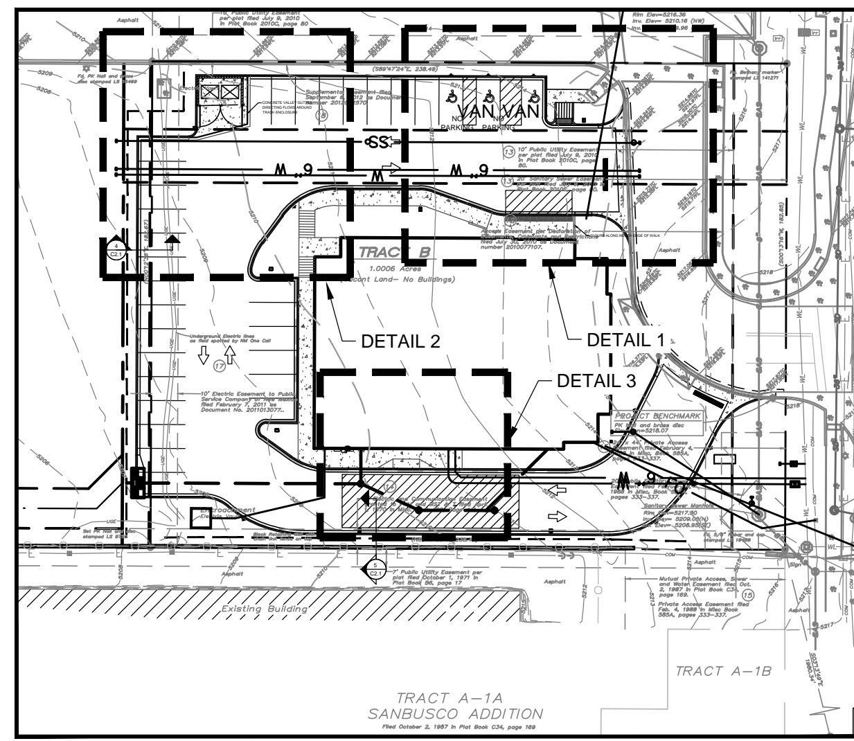
KEY MAP
