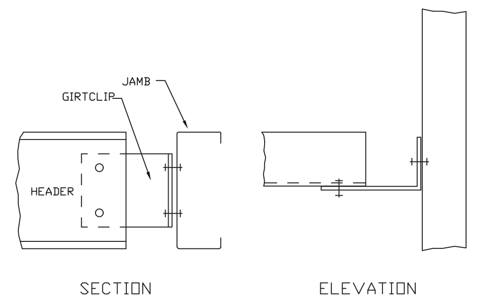
M1 HEADER TO C JAMB
