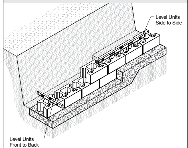
A:4 - LEVELING PAD
