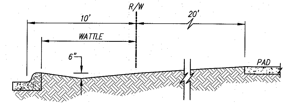
SCALE: 1"=5'
