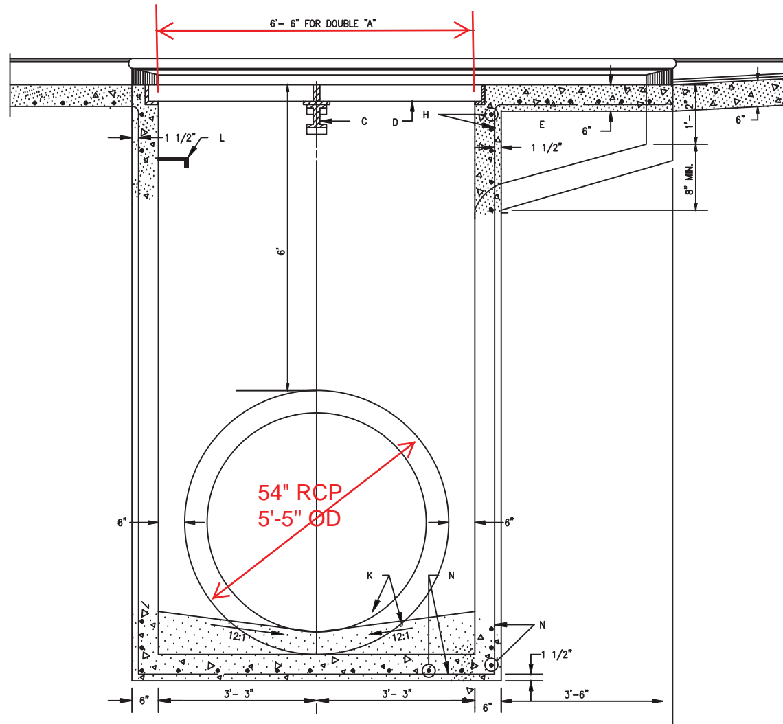
SECTION A-A
