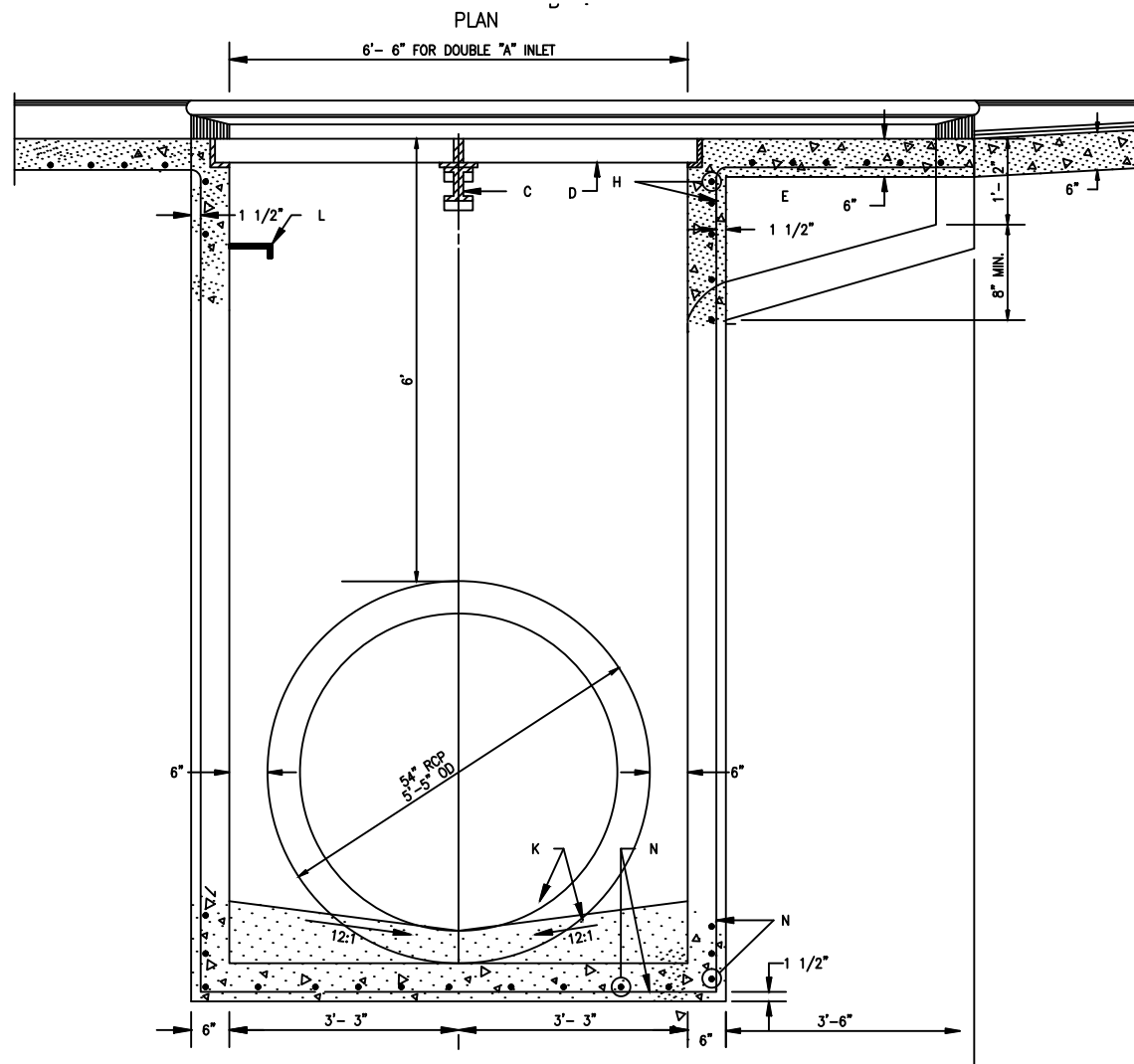
SECTION A-A
