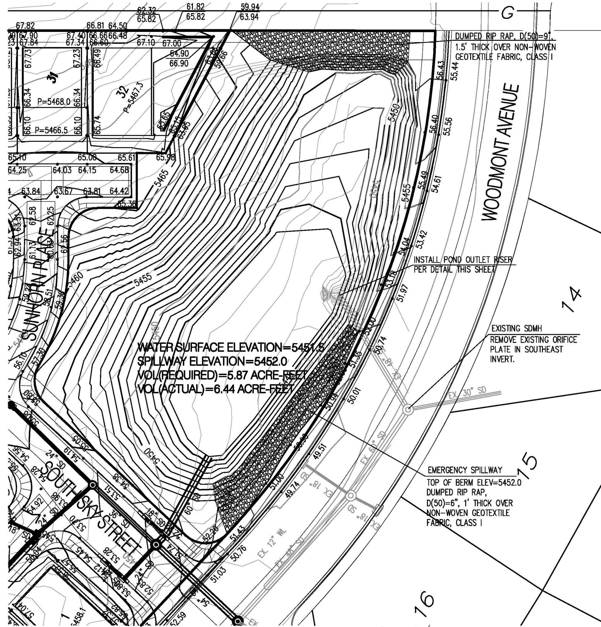
POND E SCALE: 1" = 50'
