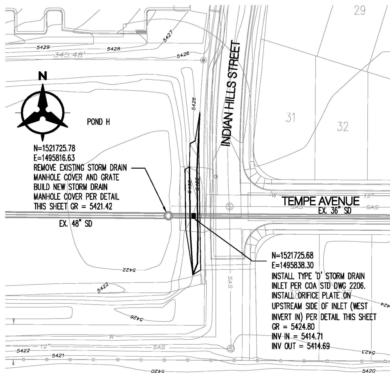
POND H OUTLET MODIFICATIONS SCALE: 1" = 50'
