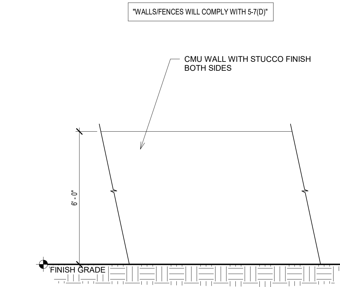
14 PERIMETER SOLID WALL SCALE: 3/8" = 1'-0"
