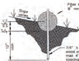
ENTRENCHMENT DETAIL N.T.S.
