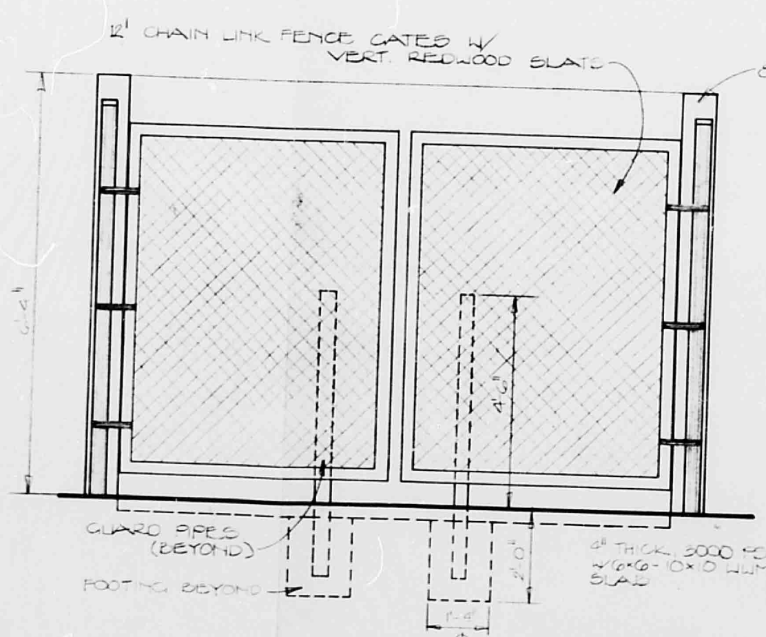
TRASH ENCLOSURE ELEVATION E SCALE: 3/8"=1'-0"
