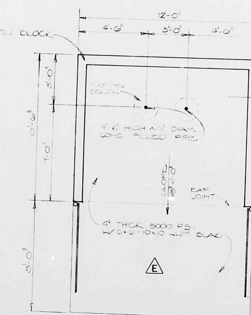
TRASH ENCLOSURE SCALE: 1/4"=1'-0"
