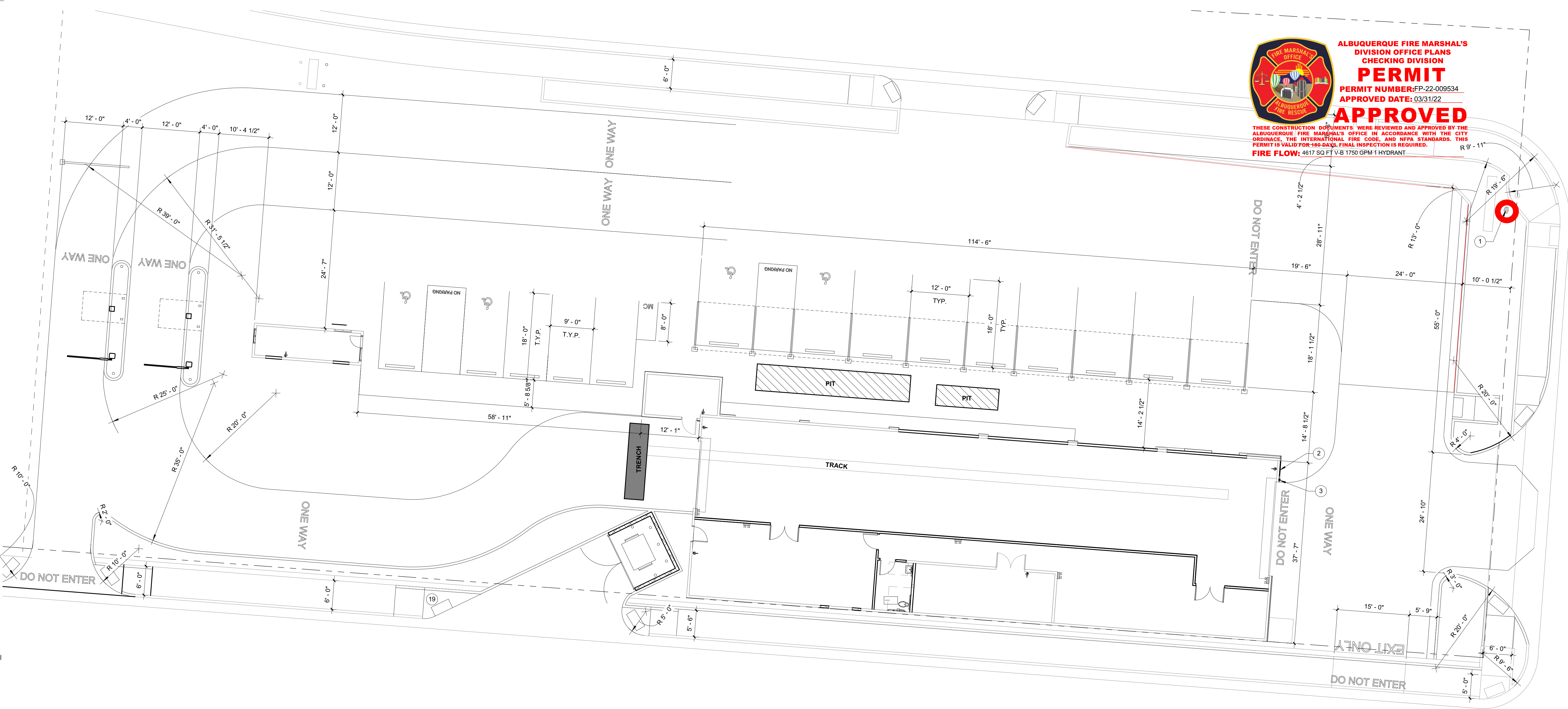
1 FIRE 1 PLAN SCALE: 1" = 10'-0"
