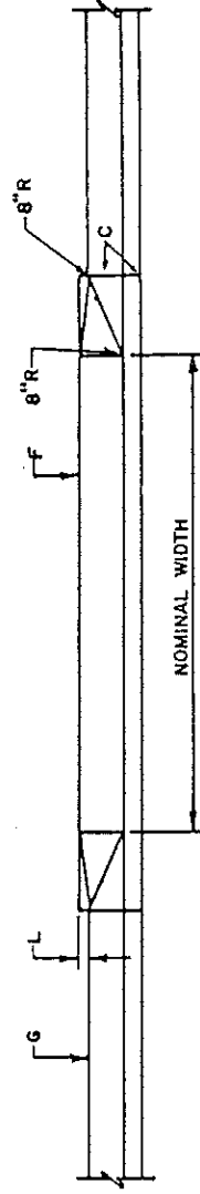
ELEVATION
