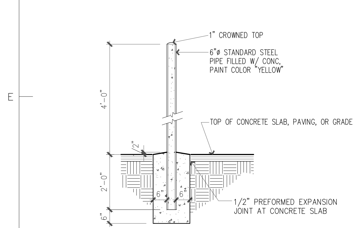
D1 STEEL PIPE BOLLARD SCALE: 1/2" = 1'-0"
