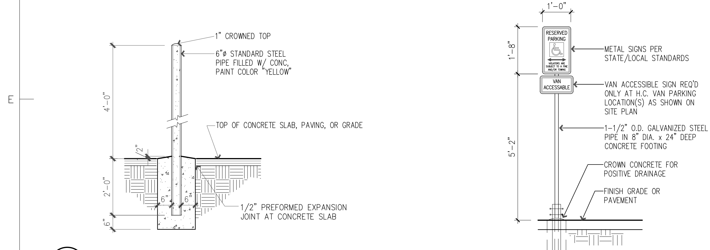
D1 STEEL PIPE BOLLARD SCALE: 1/2" = 1'-0"
