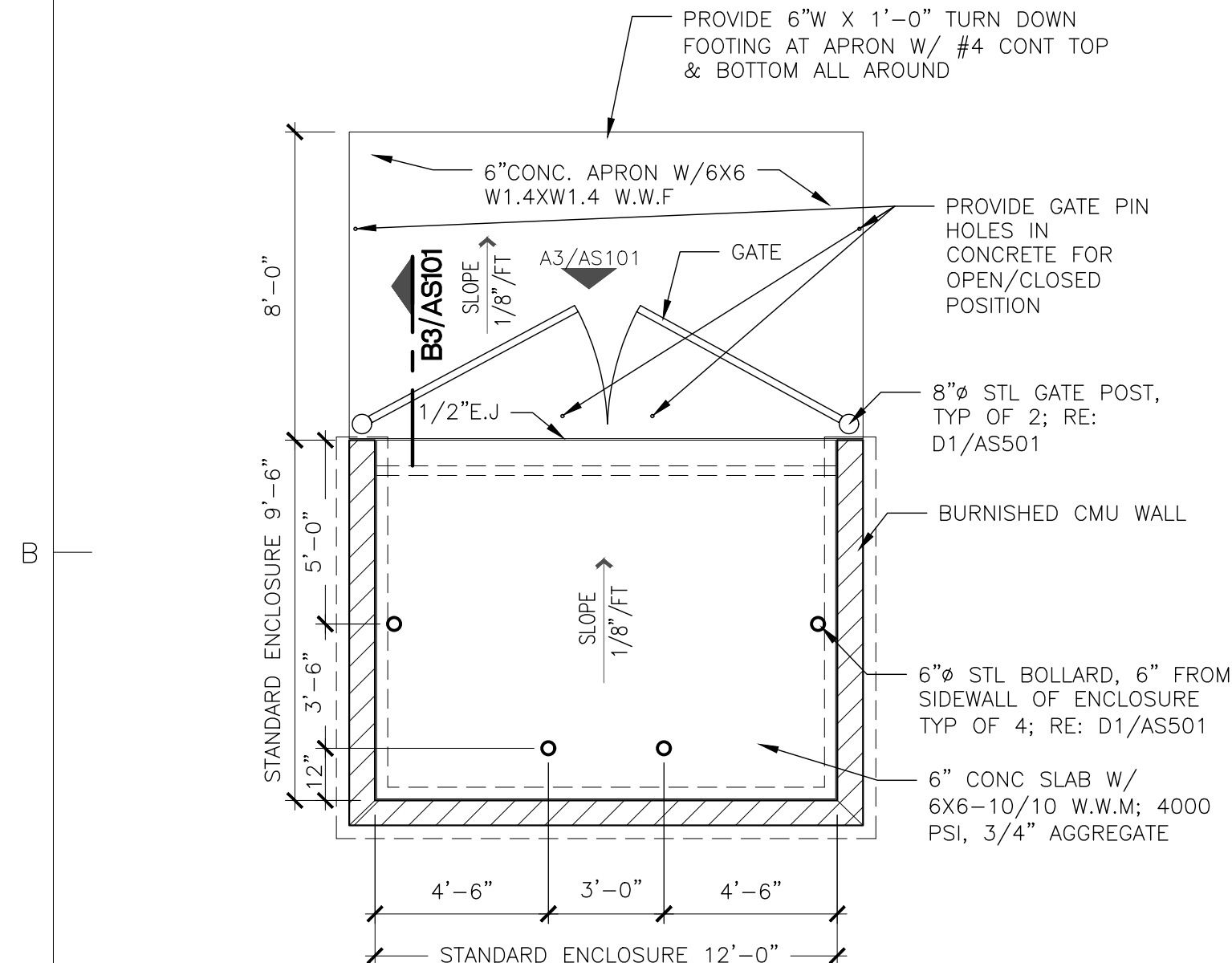
A1 TRASH ENCLOSURE PLAN SCALE: 1/4" = 1'-0"
