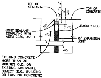
4 C7 EXPANSION JOINT (EJ) N.T.S.
