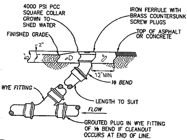
1 C7 CLEANOUT DETAILS N.T.S.
